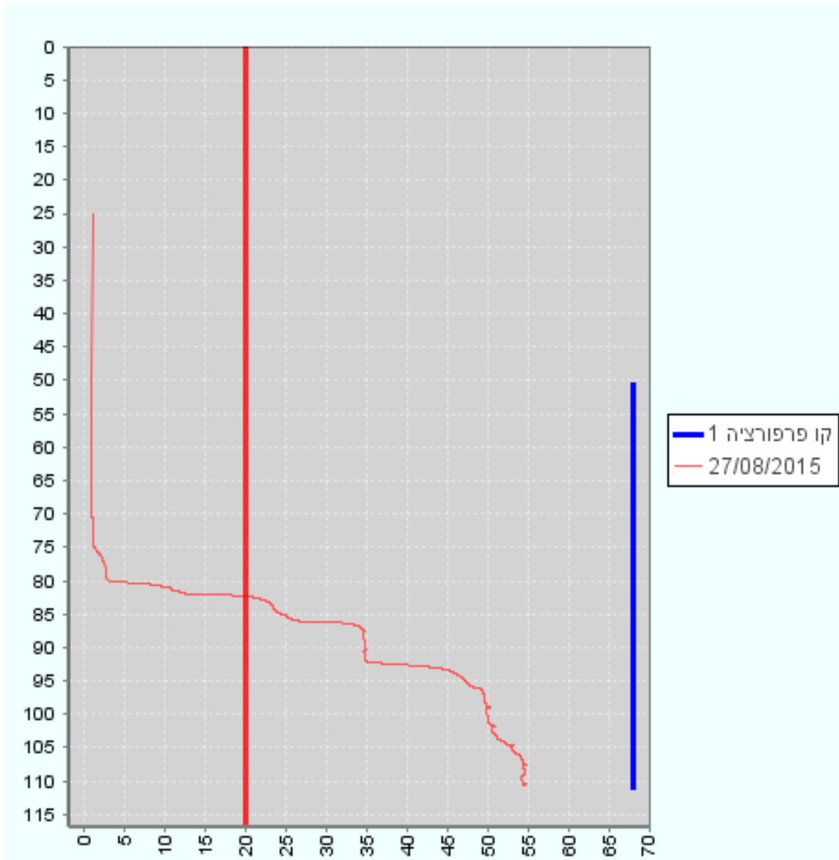
פרופיל מוליכות חשמלית של קידוח מח 104 ת2 (11510504). ציר ה-Y, עומק (מ'), ציר ה-X, מוליכות חשמלית mS/cm.
