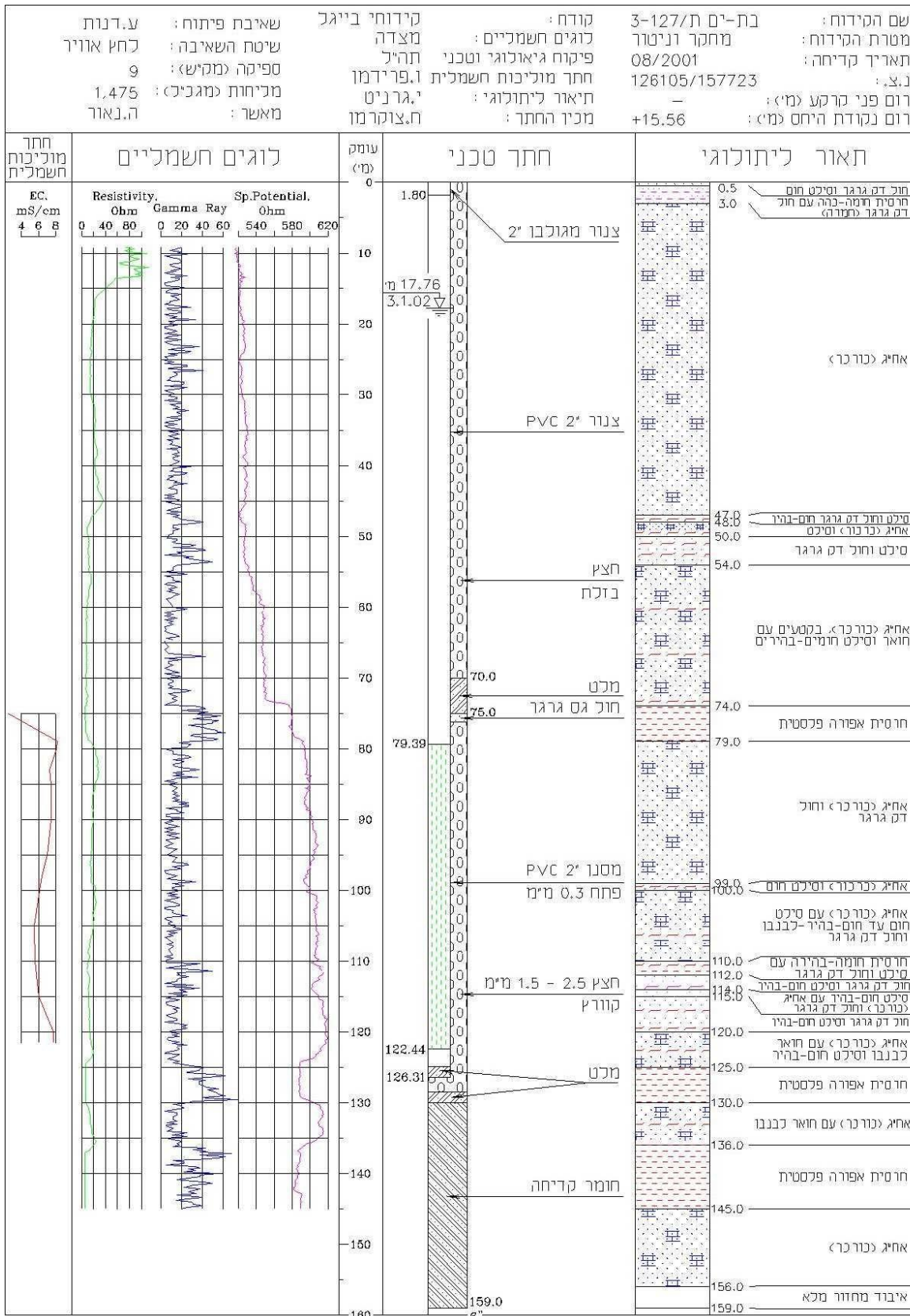
לוגים גיאופיזיים בקידוח בת ים 127 צ3 (כולל את המקטע של קידוח בת ים 127 צ4)
