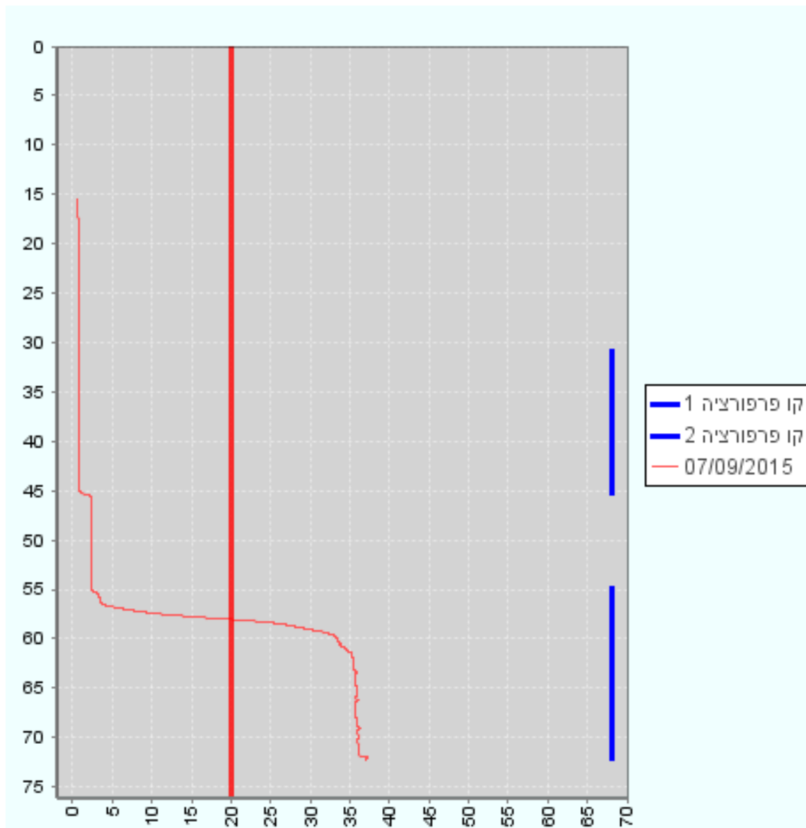
פרופיל מוליכות בקידוח בת ים 127 צ.4. ציר ה-Y, עומק (מ'). ציר ה-X, מוליכות חשמלית mS/cm.
