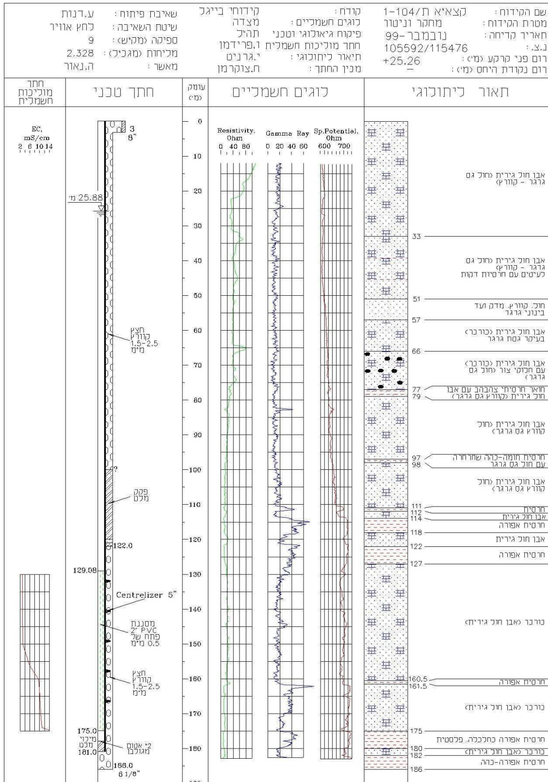
לוגים חשמליים של קידוח מח 104 ת1 (כולל את המקטע של קידוח 104 ת2)
