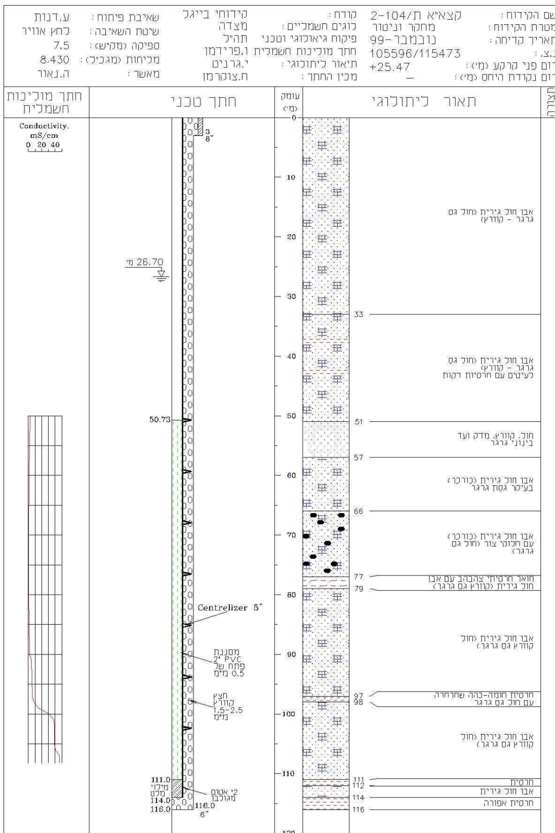
חתך גיאולוגי ומפרט טכני של קידוח מח קצאא 104 ת2 (11510504).
